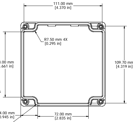
LID - INSIDE
